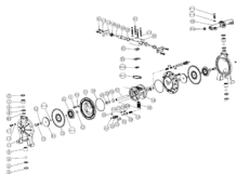
SPARE PARTS VIEW Pag. 451
