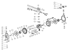
SPARE PARTS VIEW Pag. 451
